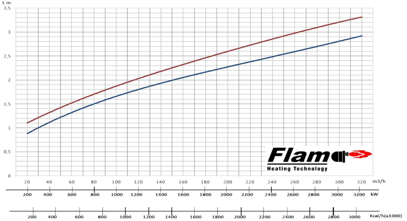
GAZ YAKIT - ALEV ÇAPI
