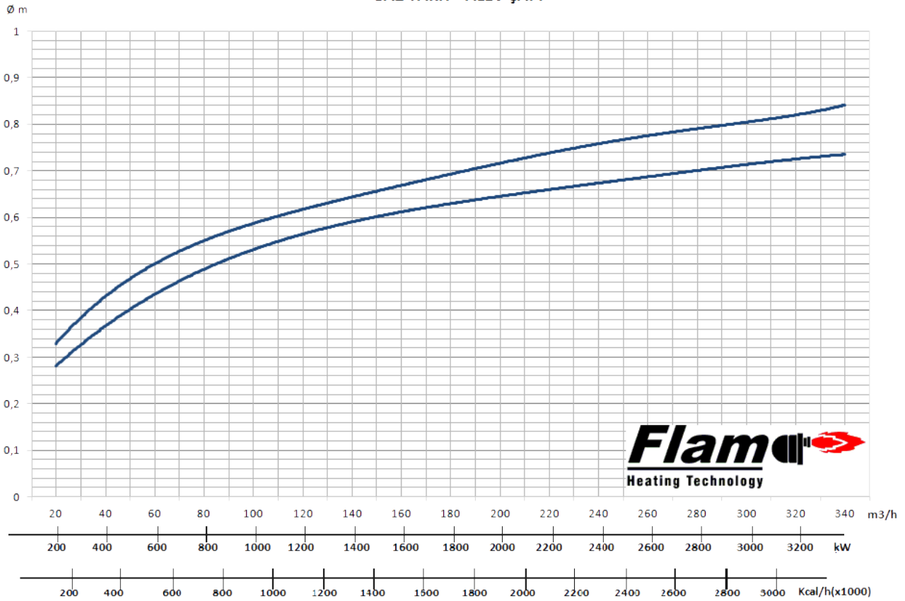
GAZ YAKIT - ALEV ÇAPI
